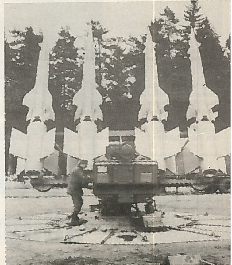
Helsingin Ilmatorjuntarykmentin ohjuskalustoon kuuluva alueilmatorjuntaohjus.
