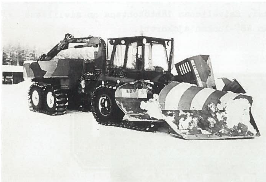
Aurausmetsätraktori Valmet Jehu
